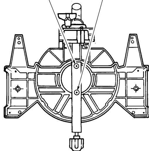
Tornillos de casquete del resorte del índice de ingletes
