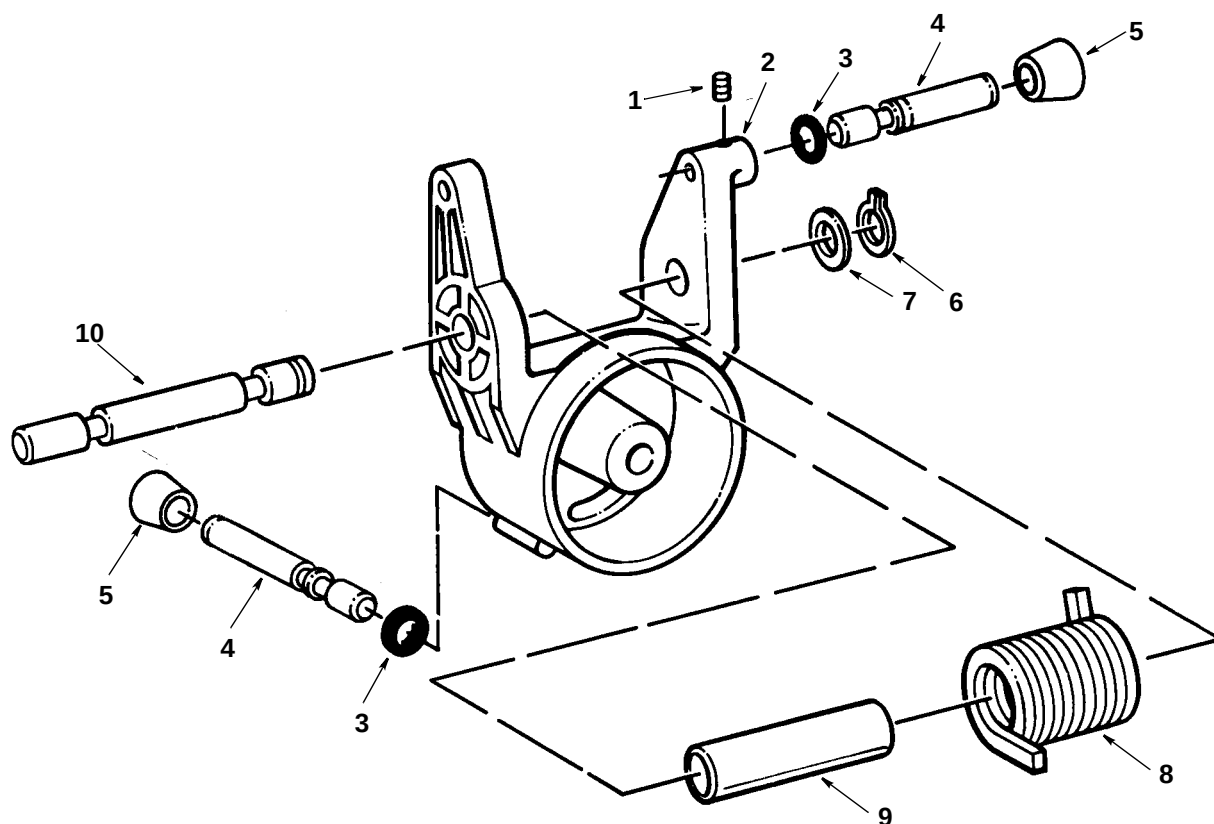
Figura 3 – Ensamblaje del pivote
