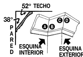
MOLDURA DE TECHO ESTANDAR DE LOS EE.UU.
