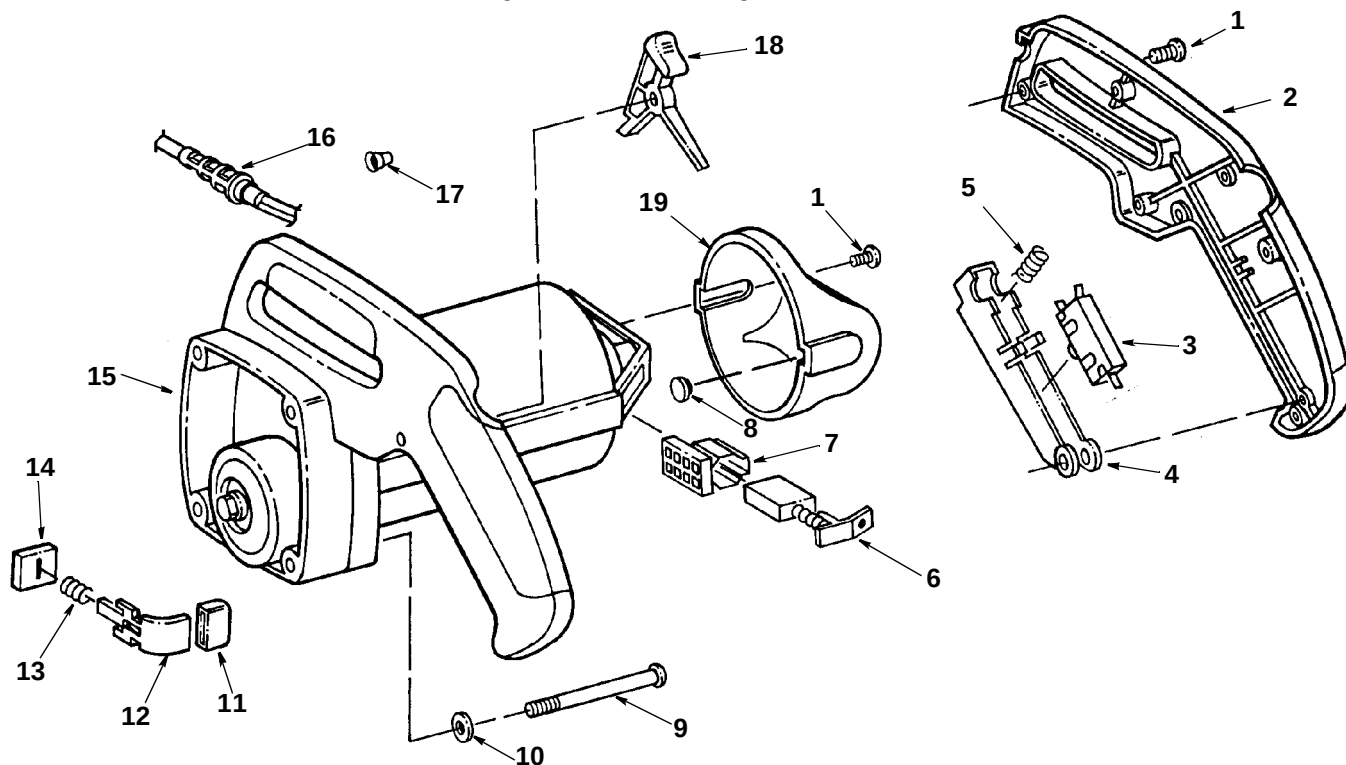
Figura 2 – Ensamblaje del motor
